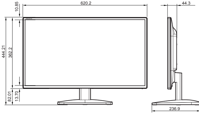
PTFBLT-27W / PTFWLT-27W 寸法図
